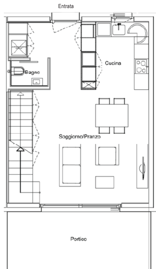
Piano Inferiore
